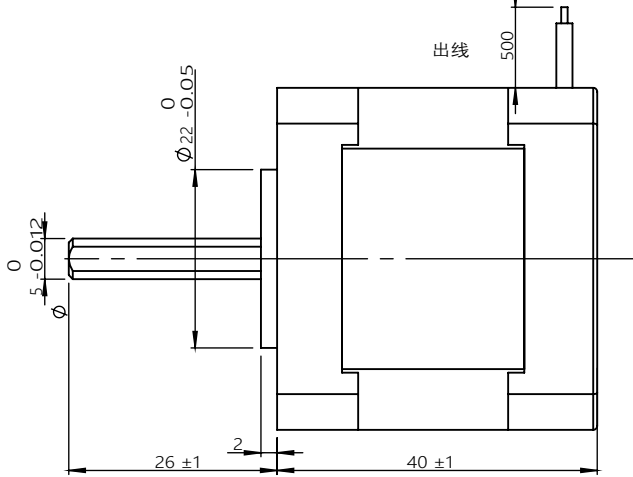
尺寸图
