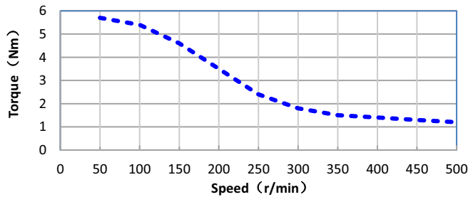
电机矩频特性曲线
