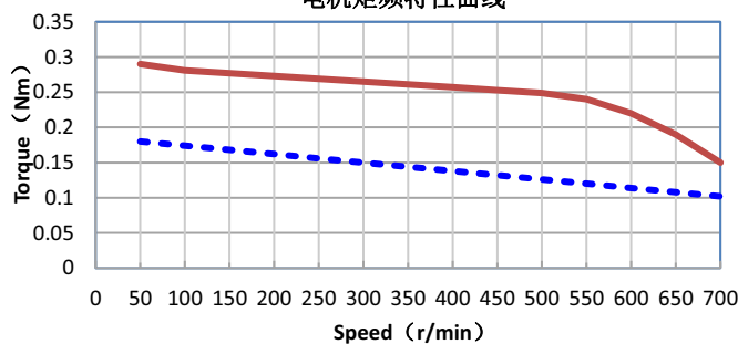
电机矩频特性曲线
