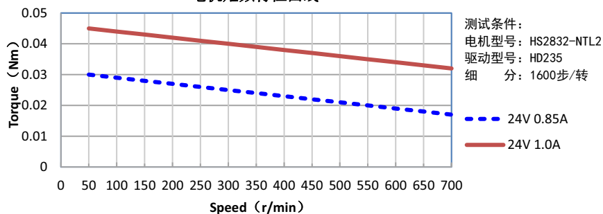
电机矩频特性曲线
