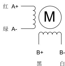
电机接线图
