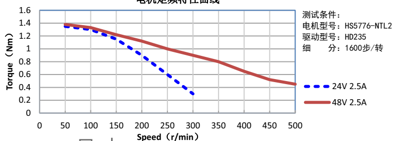
电机矩频特性曲线
